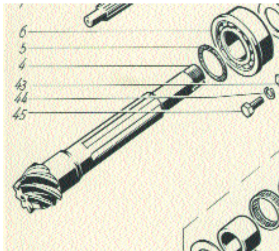
Abbildung 1: Abtriebswelle
