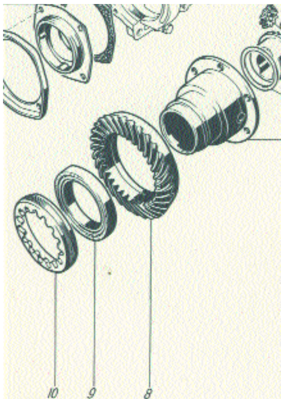
Abbildung 2: Differentialrad
